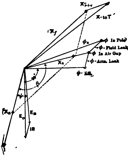
FIG. 10.—NIETHAMMER DIAGRAM.
