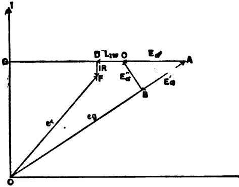
FIG. 9.—ARNOLD DIAGRAM.
