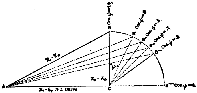
FIG. 8. — M. M. F. METHOD.
